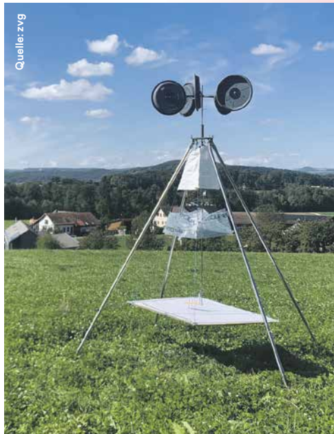
Quelle: zvg Simone Maurers Windmaschine: Das Papier liegt auf der mit dem Wind schwingenden Platte.
